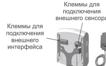
С внешним проводным интерфейсом и выносным сенсором (металлический кронштейн)
