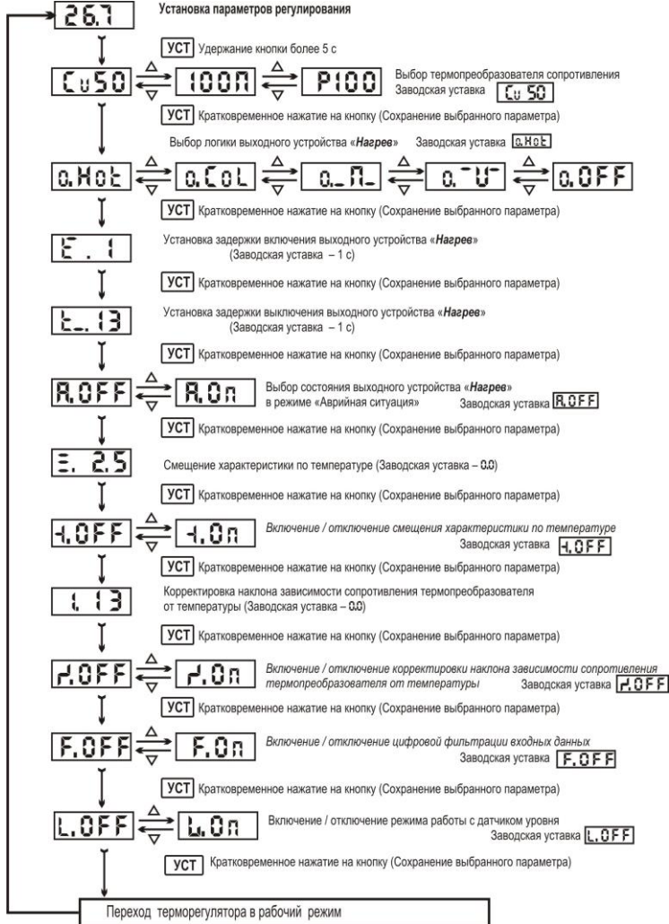
Рисунок 5 – Алгоритм программирования терморегулятора PATAP-02M.TC
